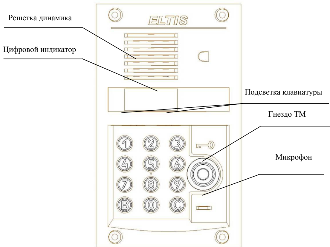
Рис.1 Внешний вид со стороны лицевой панели блока вызова DP300-TD22.
